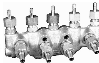
Zawory trójdrogowe MEZ-10 i pięciodrogowe MEZ-11
