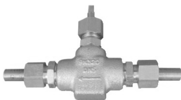
Zawory jednodrogowe MEZ-12 i manometryczne MEZ-15
