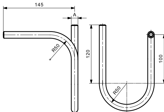
Rurka typu UB
