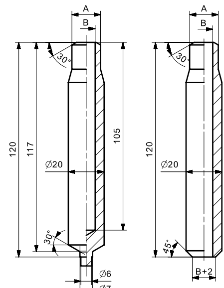
Króciec otwarty
