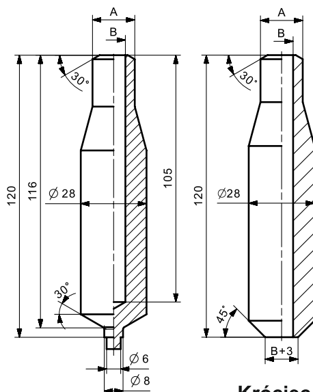
Króciec ślepy
