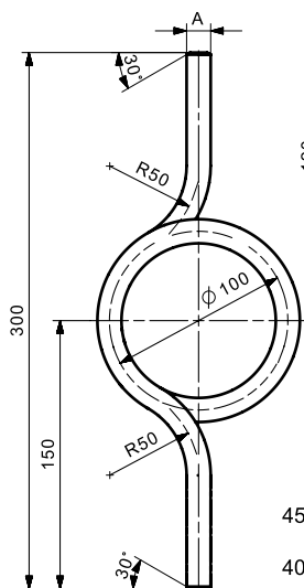
Rurka typu P
