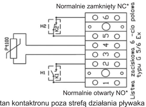
Schemat połączeń
